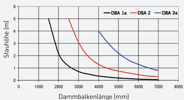
Dammbalken bei einer Biegung von M= 1/150 ; größere Feldweiten oder Höhen auf Anfrage
